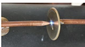
Paul stelt de afstand van de vonkenbrug in
