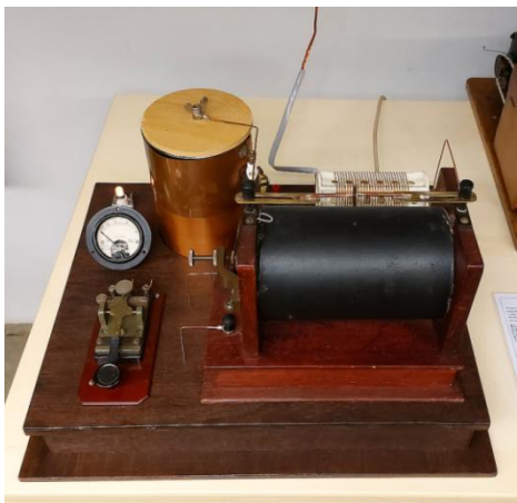
De complete zender. In de expositie is er voor de veiligheid een plexiglas kap over de zender geplaatst.
