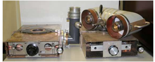
Klystron kamers en een flinke U-link
